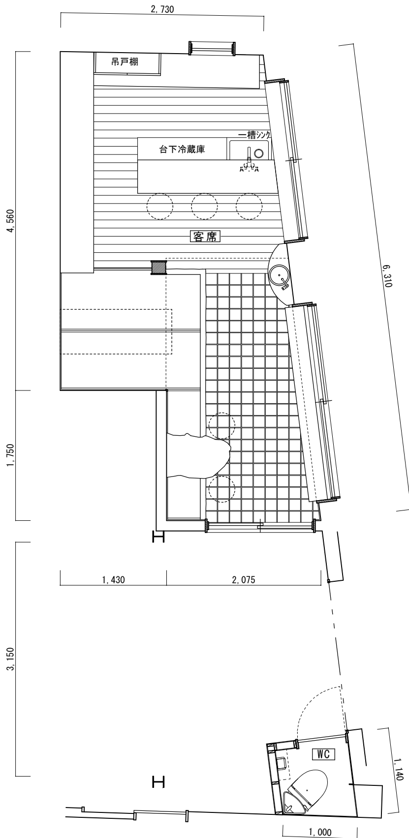
平面詳細図 S=1/50
